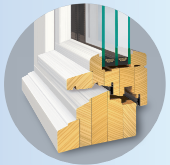
Wasserschinkel auf Flügel und Blendrahmen
